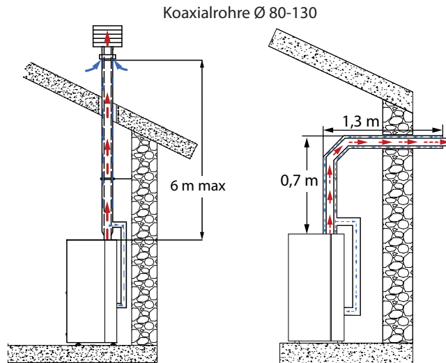
Koaxialinstallation Typ „e“ und „f“ mit Zubehör (sofern vorhanden) *
