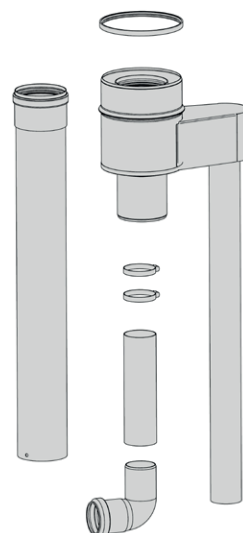
OPTIONALES ZUBEHÖR (KOAXIALES KIT) OBERER KOAXIALER RAUCHAUSLASS*
