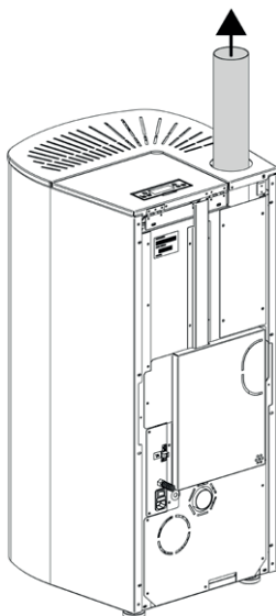
OPTIONALES ZUBEHÖR (Verlängerung) OBERER RAUCHAUSLASS
