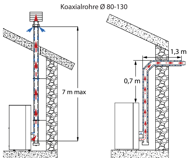
Koaxiale Installation Typ "c" (wo vorgesehen) *
