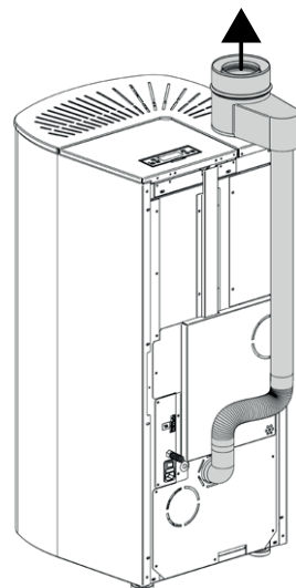
OPTIONALES ZUBEHÖR (KOAXIALES KIT) OBERER KOAXIALER RAUCHAUSLASS*
