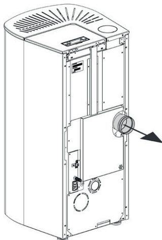
OPTIONALES ZUBEHÖR (90°-Bogen) HINTERER RAUCHAUSLASS
